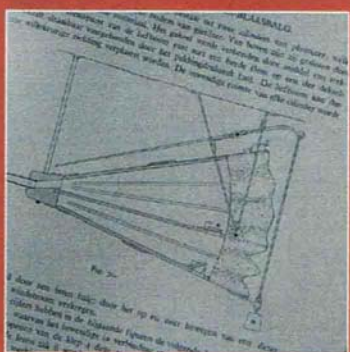
Een pagina uit het Handboek voor Smeden met daarop een tekening van één van 'onze' blaasbalgen. De werking ervan is duidelijk af te lezen.
